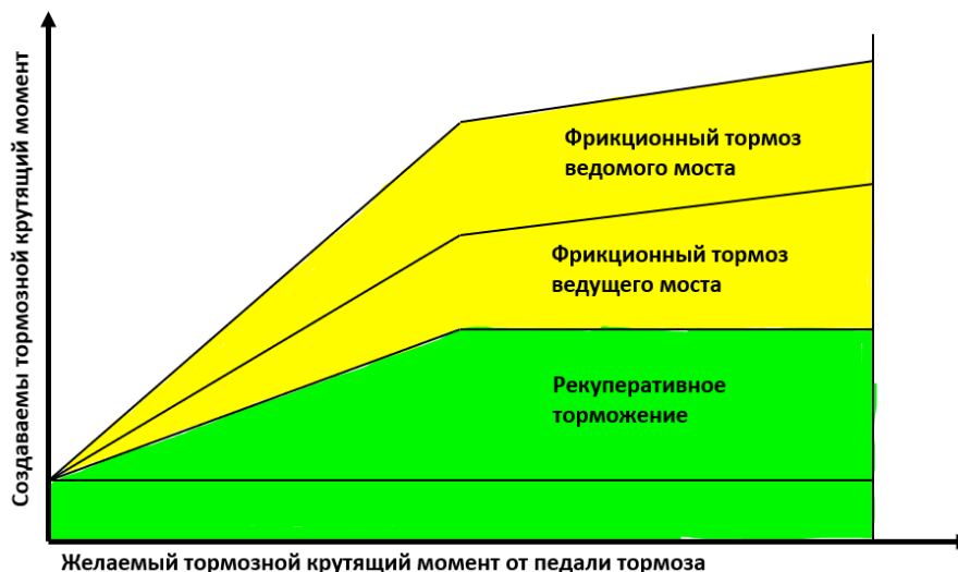
Рис. 8 Параллельное рекуперативное торможение.
