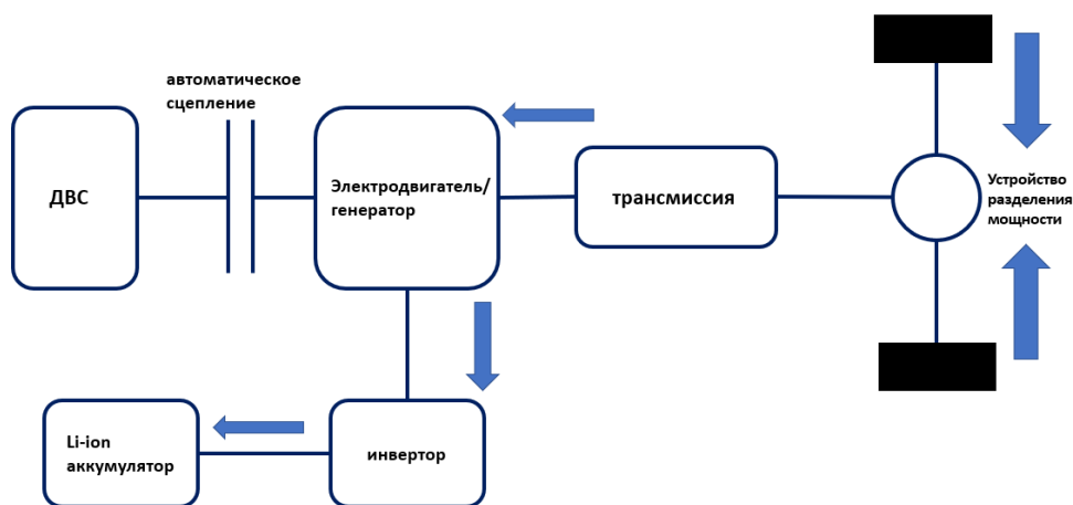
Рис. 6 Схема рекуперативного торможения.
