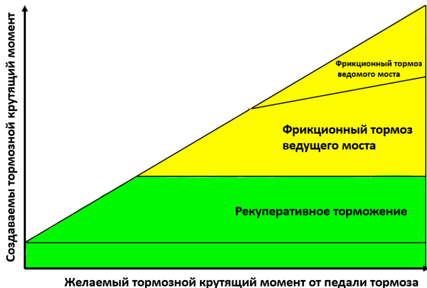
Рис. 7 Последовательное рекуперативное торможение.
